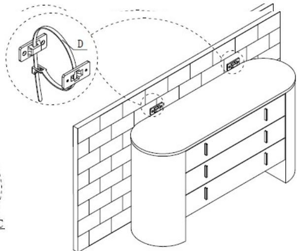
Paso 5 Step 5
